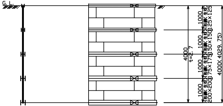
1-1 断面図 S=1/40
