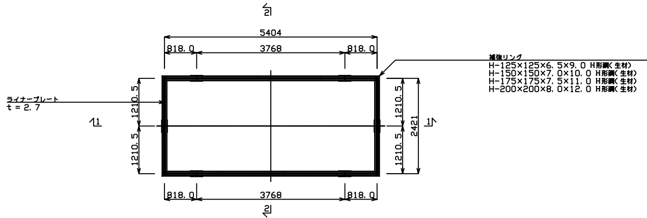
平面図 S=1/40
