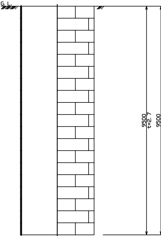
1-1 断面図 S=1/40
