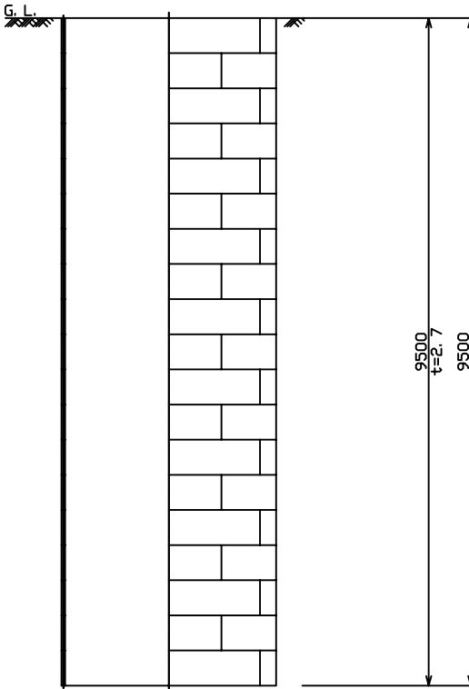
2-2 断面図 S=1/40
